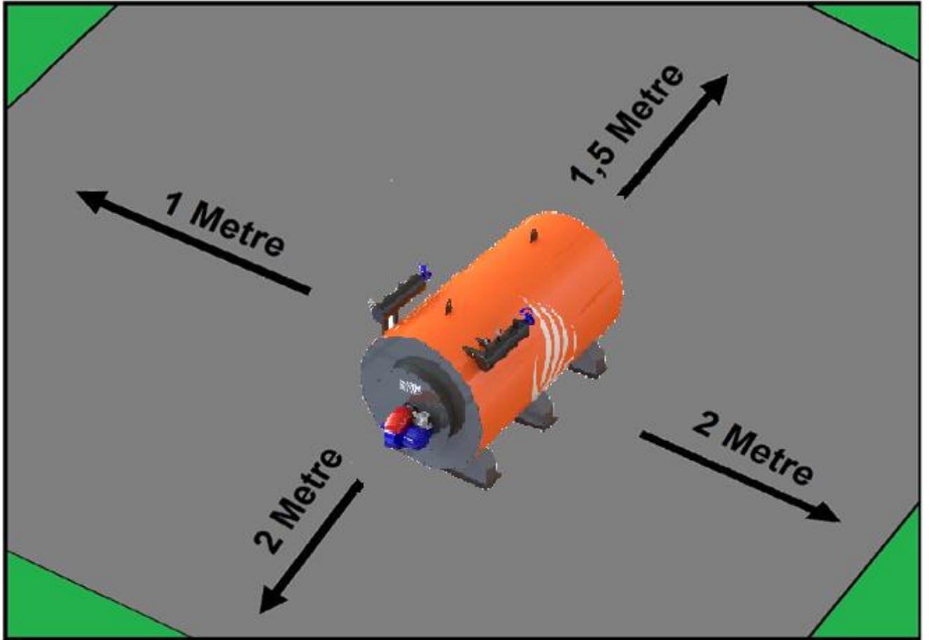
Katı Yakıtlı Kızgın Yağ Kazanı Yerleşimi Temsili Çizimi
